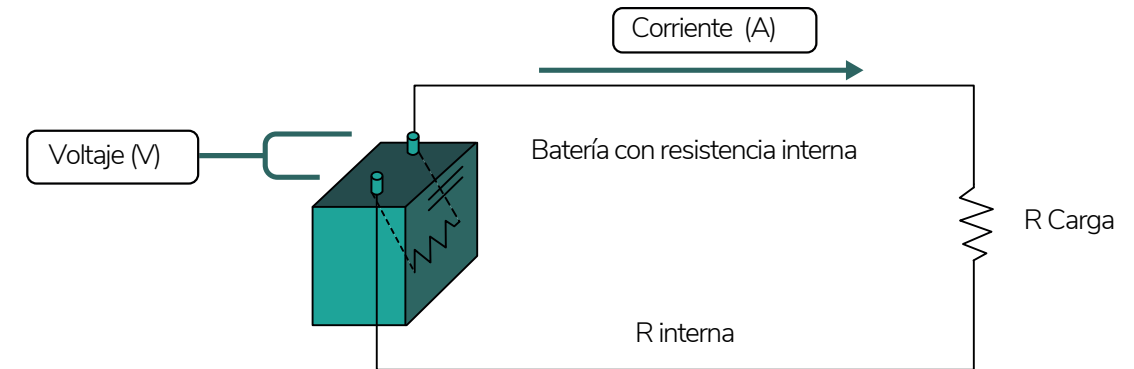
Figura 8 ▶ Circuito eléctrico de una batería
