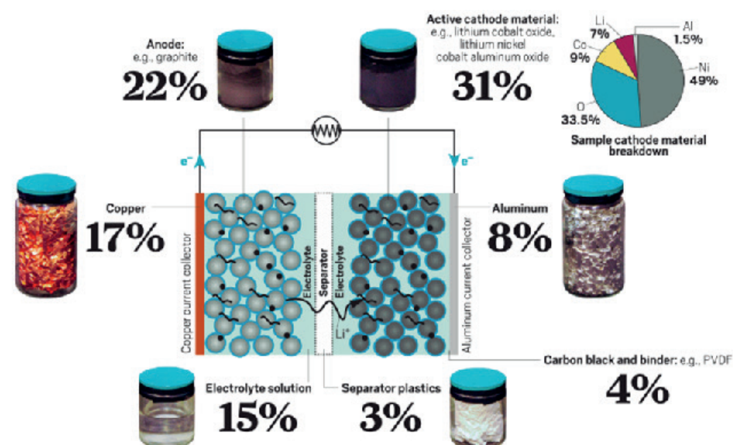
Figura 20 ▶ Componentes internos de una batería de iones de litio
