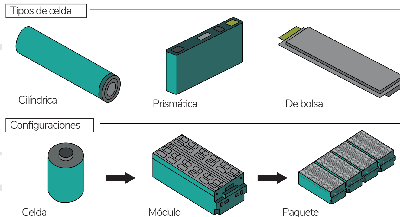
Figura 4 ▶ Tipos de celdas y configuraciones más comunes de las baterías de iones de litio utilizadas en vehículos eléctricos
