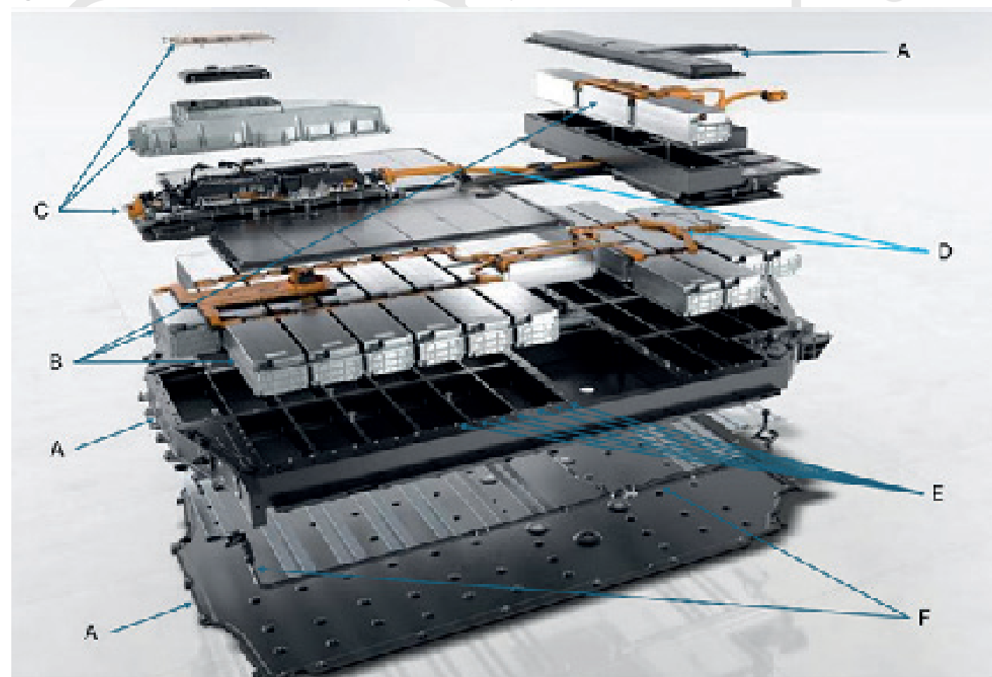
Figura 18 ▶ Partes de una batería de iones de litio con potencial de aprovechamiento
